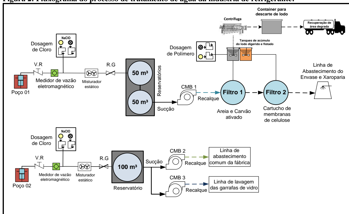
Figura 2: Fluxograma do processo de tratamento de água da indústria de refrigerante.
