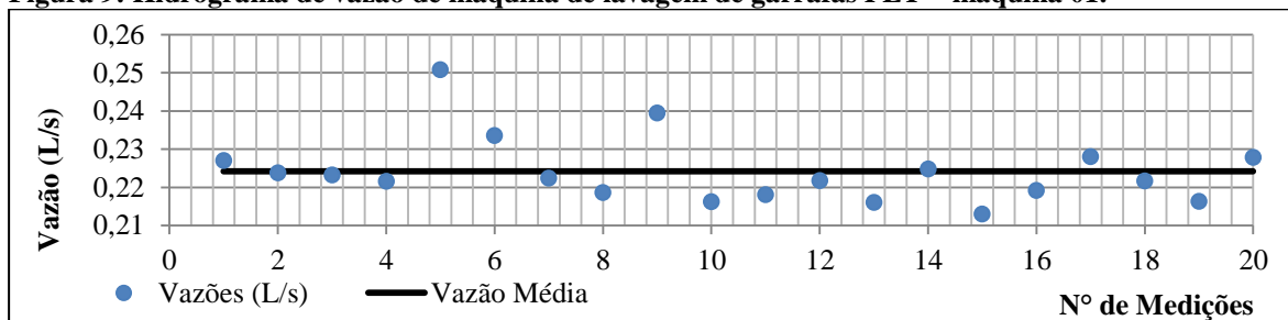
Figura 9: Hidrograma de vazão de máquina de lavagem de garrafas PET – máquina 01.
