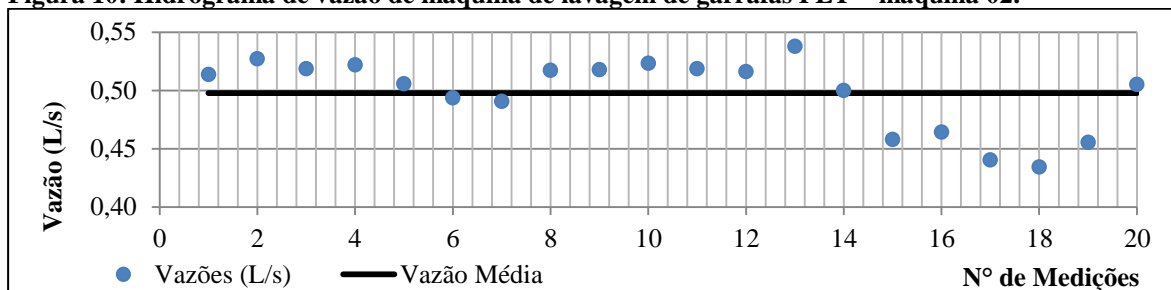
Figura 10: Hidrograma de vazão de máquina de lavagem de garrafas PET – máquina 02.
