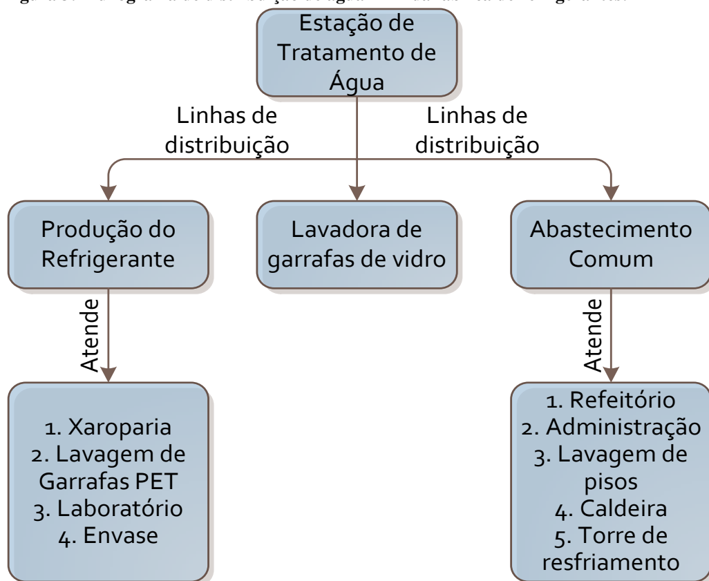
Figura 3: Fluxograma de distribuição de água ETA da fábrica de refrigerantes.
