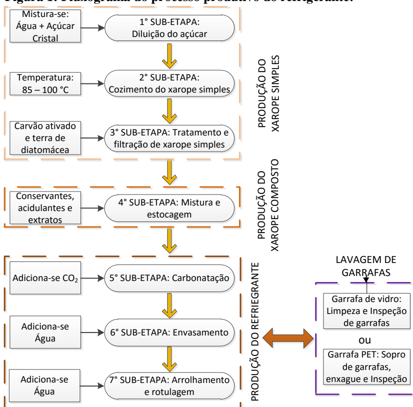
Figura 1: Fluxograma do processo produtivo do refrigerante.
