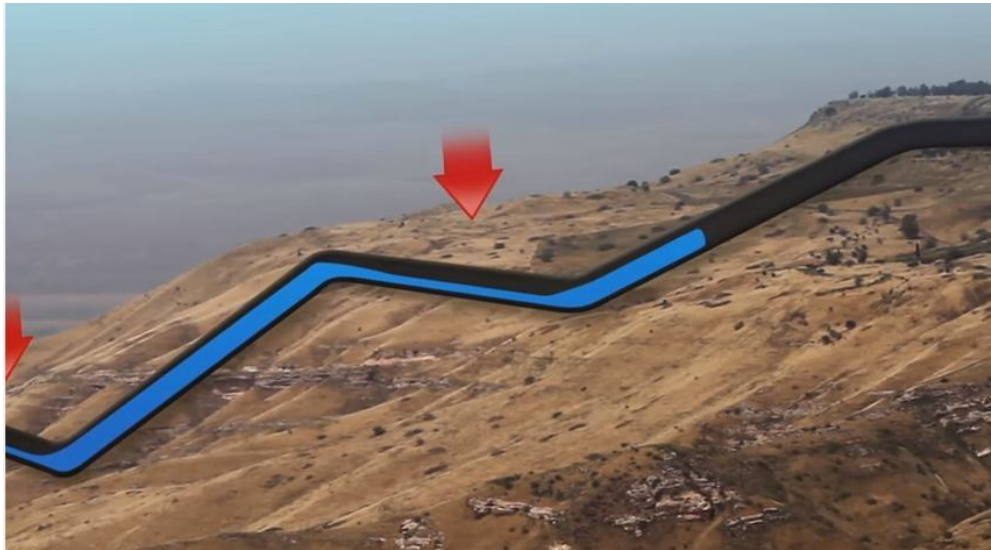
Figura 1: Imagem de uma rede de abastecimento sem válvula ventosa. Trecho da tubulação fica sem preenchimento, o que causa um maior esforço a passagem da água.
