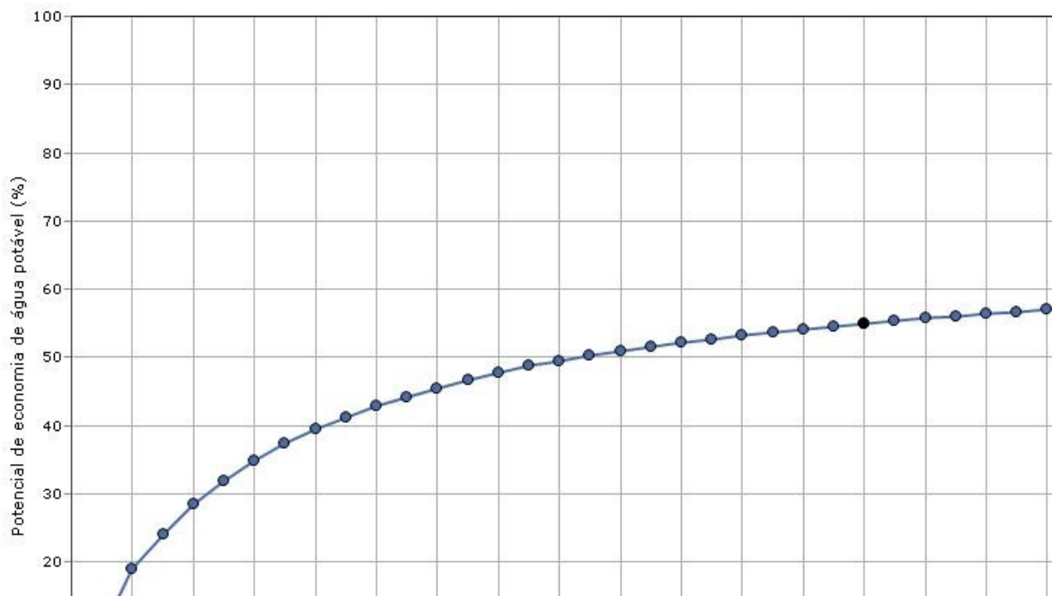
Figura 1: Relação entre o volume do reservatório inferior e o potencial de economia de água potável.
