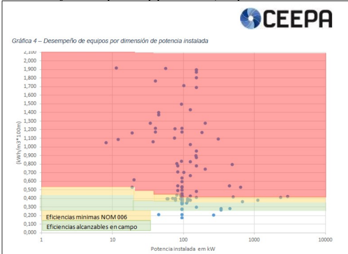
Figura 2: Desempenho dos equipamentos em função da potência instalada
